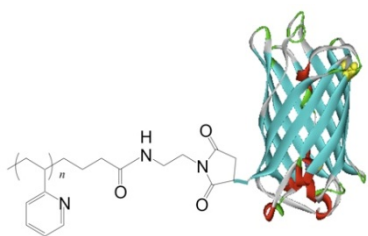
図1 GFP-p2VPの構造
