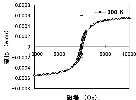
図1. カリウムドープポリマーのMH曲線、試料重量25.8 mg.
