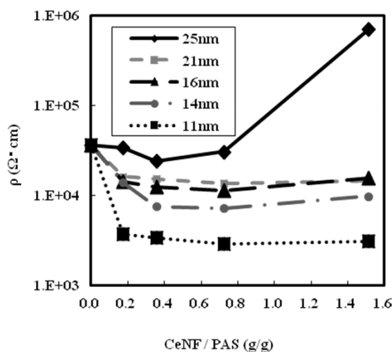
図1 PAS/PEs/CeNF 複合材料の体積抵抗率
